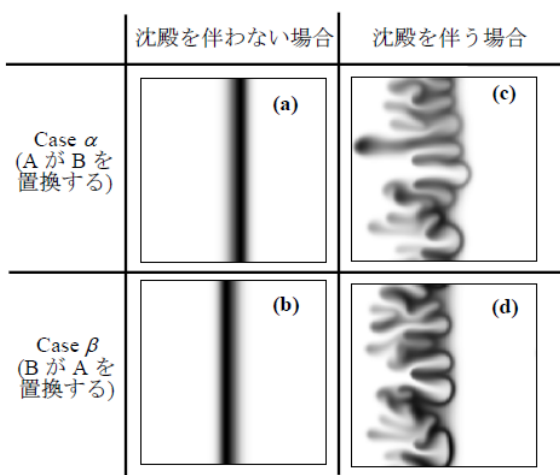
図3 化学反応を伴う置換の数値解析結果 置換の方向は左から右。生成物分布をグレースケールで表している。この数値計算では、化学種 A の拡散係数は化学種 B の拡散係数より 4 倍大きいとしている。A が B を置換する場合の方が、生成物が広く分布する。
