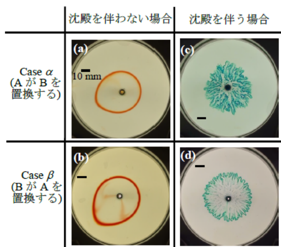
図2 化学反応を伴う置換パターン 置換開始 840 s 後。生成物が呈色している。(a)(b)沈殿を伴わない場合、流体力学的に安定な円形な置換パターンとなり、化学種 A が化学種 B を置換する場合も、B が A を置換する場合も、置換パターンは変わらない。(c)(d)沈殿を伴う場合、流体力学的不安定となり、Fingering (指状) パターンとなる。A が B を置換する場合と B が A を置換する場合で Fingering パターンの特徴は異なり、A が B を置換する場合、生成物が広く分布する。
